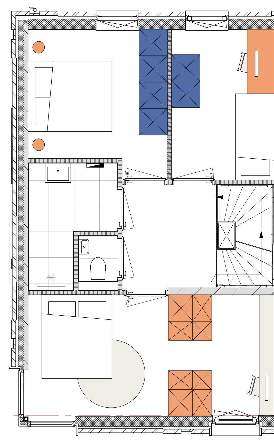
eerste verdieping
