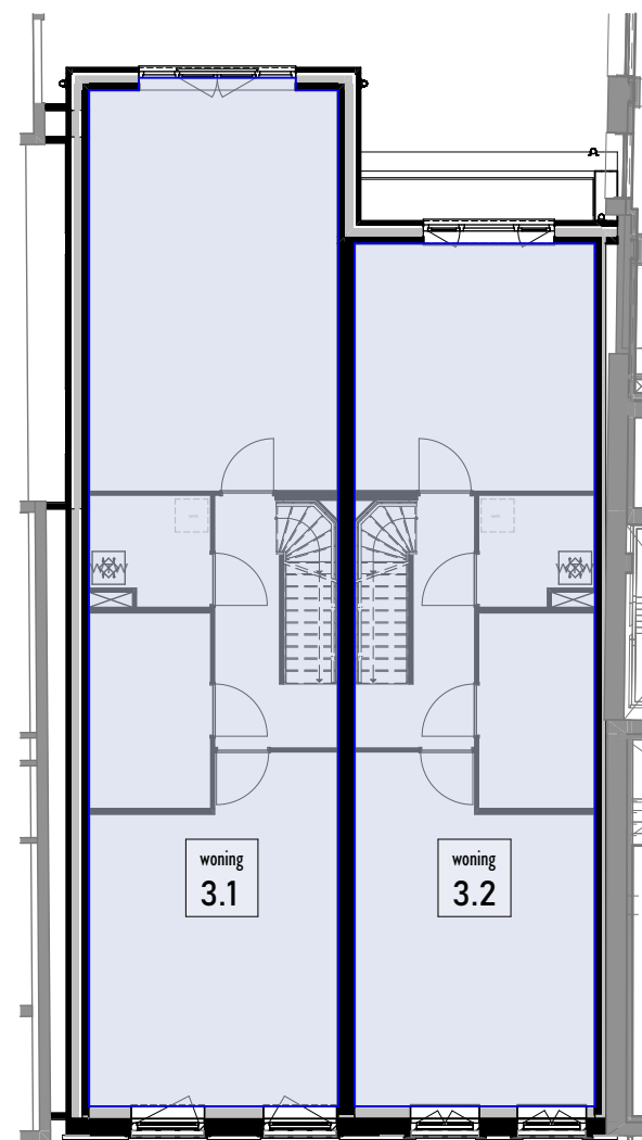
eerste verdieping
