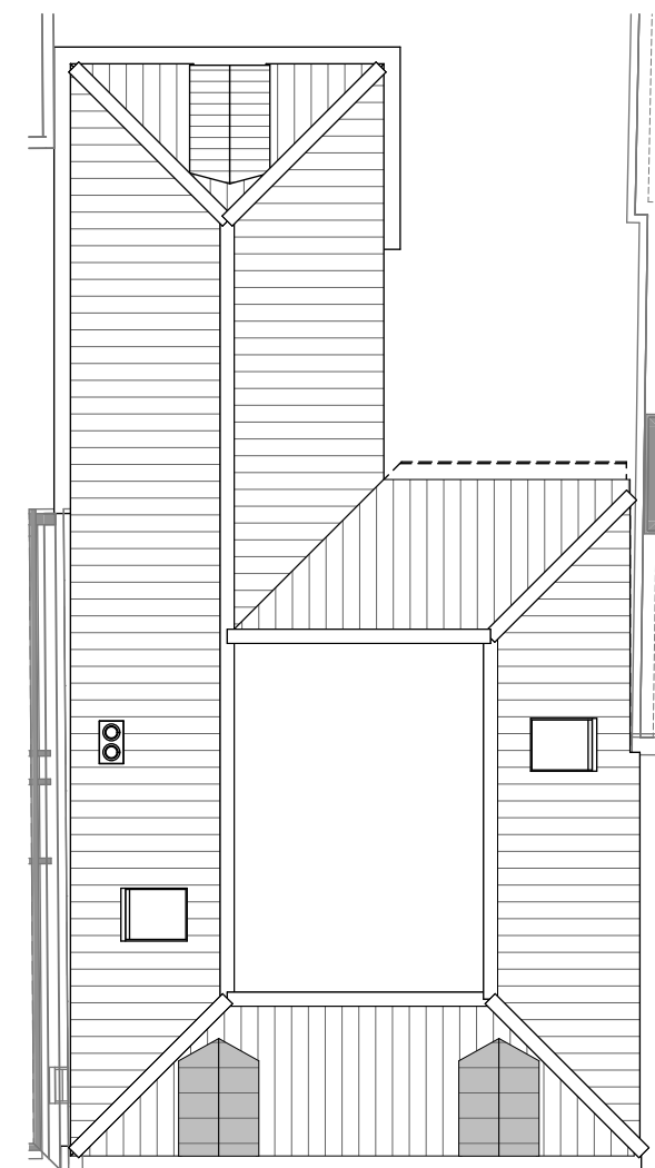
dakaanzicht
