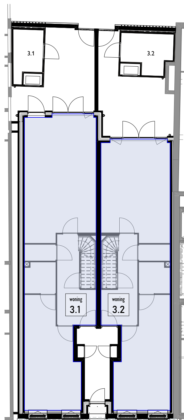
begane grond
